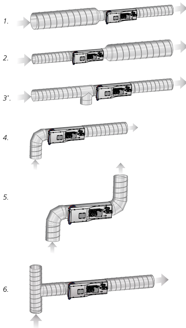
Figur 5. Krav til rett strekning sirkulære kanaler.
