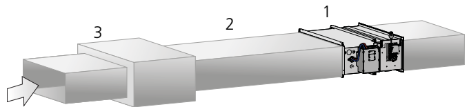
Figur 8. Krav til rett strekning for rektangulær WISE Damper og lyddemper med baffel. Montering med rett strekning gjelder både til- og avtrekksluft.
