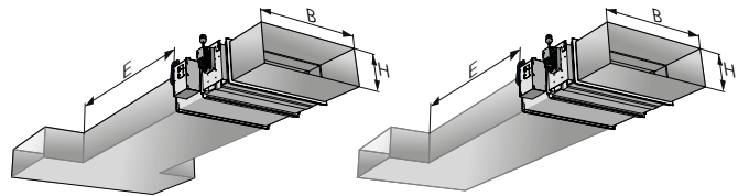
Figur 7. Krav til rett strekning for rektangulære kanaler.
