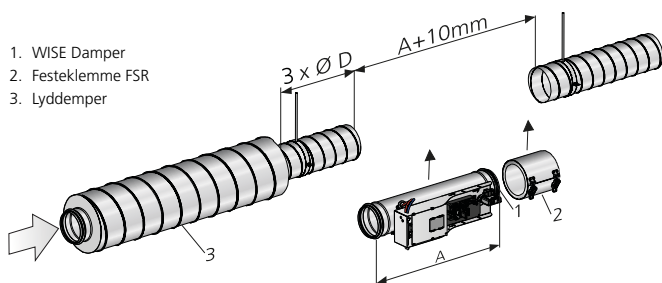
Figur 3. Krav til rett strekning 3 x Ø ved lyddemper med baffel eller akustisk kjerne.
