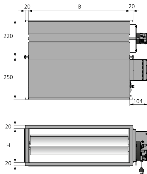
Figur 9. Mål, WISE Damper rektangulær, WISE Damper rektangulær med fjærtilbakestilling.
