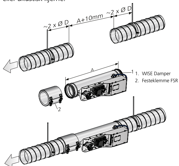
Figur 4. Installasjon i kanalsystemet. Kanalene må festes i bygningsstammen på hver side av WISE Damper.
