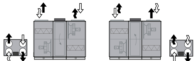
Ventilatorstand 1 ingesteld als inlaatlucht (inspectiezijde links)
