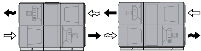
Ventilatorstand 1 ingesteld als uitlaatlucht (inspectiezijde rechts)
