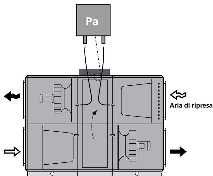
Principio di collegamento per la funzione di sbrinatoria con sensore di pressione separato.
