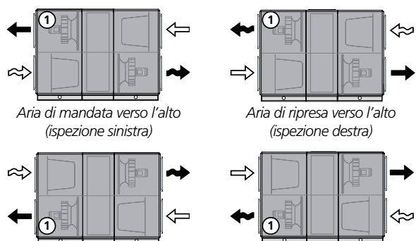
Aria di mandata verso l'alto (ispezione sinistra) Aria di mandata verso il basso (ispezione sinistra). Non RX taglie 004-008 in alloggiamento comune.
