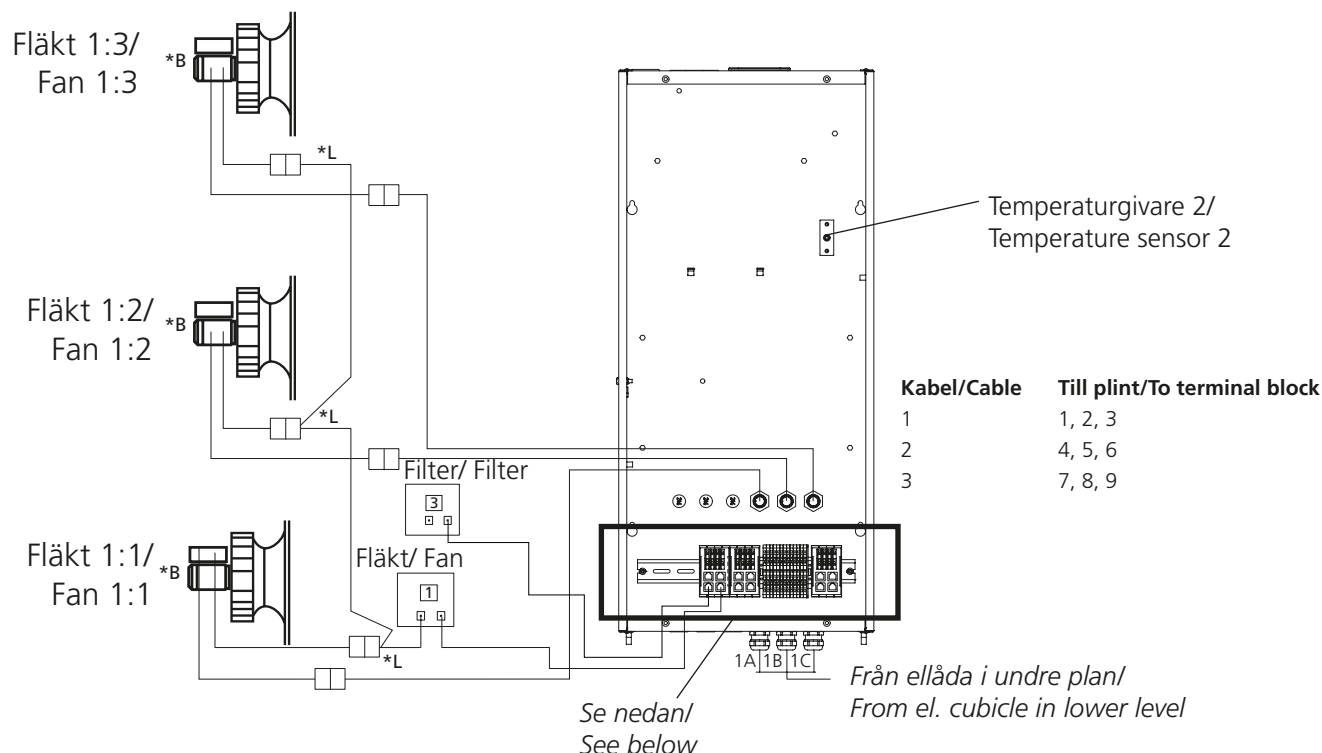
Tilluft i övre plan med fläkt till vänster om visad ellåda/ Supply air in upper level, fan to the left of shown el. cubicle
