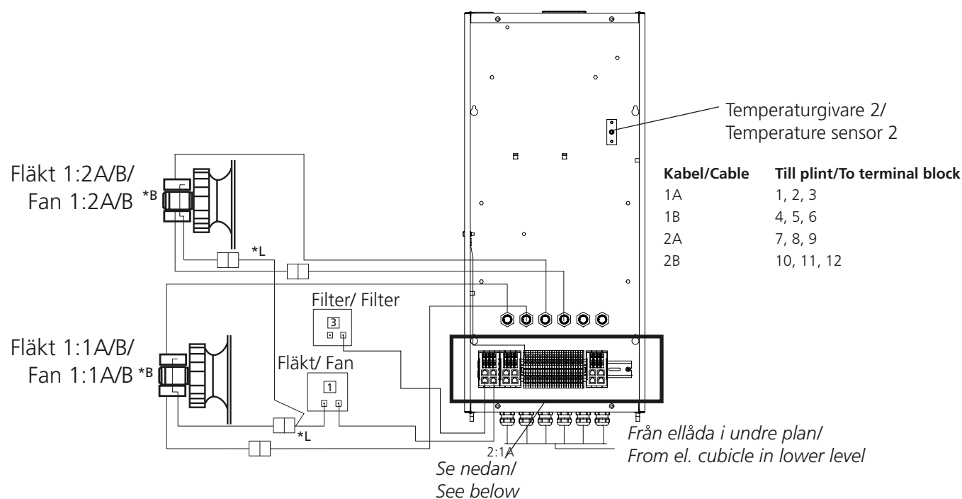
Tilluft i övre plan med fläkt till vänster om visad ellåda/ Supply air in upper level, fan to the left of shown el. cubicle
