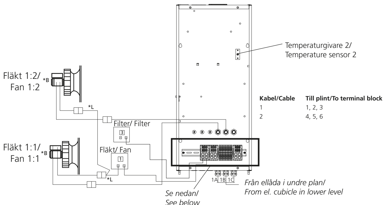
Tilluft i övre plan med fläkt till vänster om visad ellåda/ Supply air in upper level, fan to the left of shown el. cubicle
