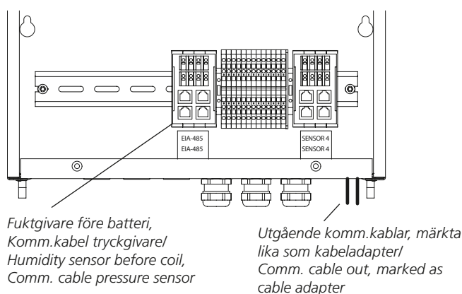
Frånluft i övre plan med fläkt till höger om visad ellåda/ Exhaust air in upper level, fan to the right of shown el. cubicle
