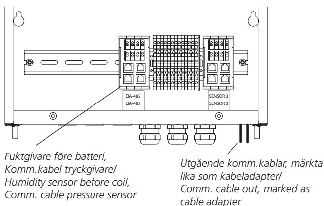
Frånluft i övre plan med fläkt till vänster om visad ellåda/ Exhaust air in upper level, fan to the left of shown el. cubicle
