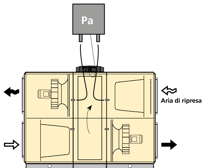
Principio di collegamento per la funzione di sbrinatura con sensore di pressione separato.
