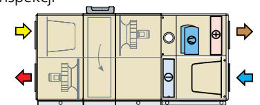
Chłodnica w dolnej części agregatu chłodniczego COOL DX Centrala GOLD - wariant 2
