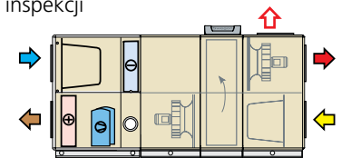
Chłodnica w górnej części agregatu chłodniczego COOL DX Centrala GOLD - wariant 2
