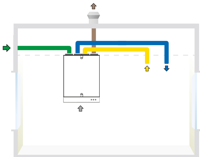
CASA R3 R, raccordements de gaines et hotte reliées au bas de l'unité de ventilation.
