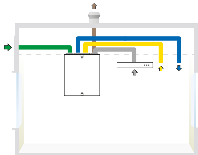
CASA R3 R, raccords de conduits et hotte raccordée au raccord de conduit de cuisine au-dessus de l'unité de ventilation.
