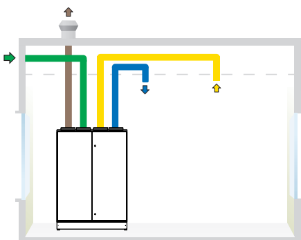
Kanaltilkoblinger på W9 L.
