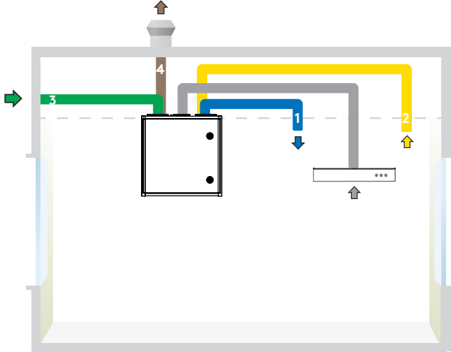
CASA R5 L, Kanalanschlüsse und Dunstabzugshaube angeschlossen am Küchenkanalanschluss des Lüftungsgeräts.
