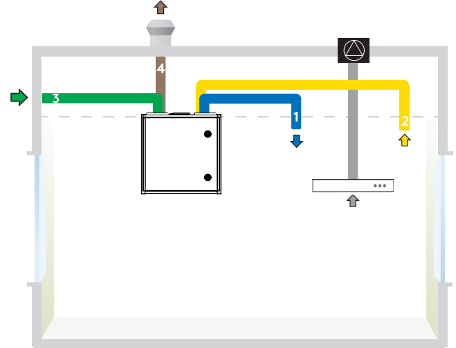
CASA R5 L, Kanalanschlüsse und Dunstabzugshaube angeschlossen an einem externen Deckenventilator.
