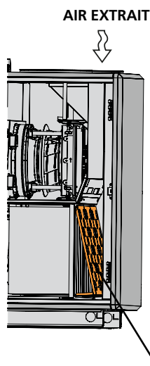
Plaque d'équilibrage Accrocher les plaques d'équilibrage sur le guide du filtre supérieur, puis enfoncer les plaques d'équilibrage vers le bas pour qu'elle se fixe dans le guide inférieur.
