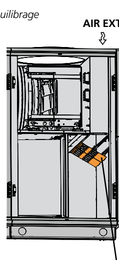
Plaque d'équilibrage Accrocher la plaque d'équilibrage dans l'encoche du côté du filtre. Soulever la plaque d'équilibrage vers le caisson de la CTA et l'accrocher dans l'encoche.
