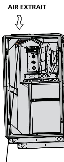
Plaques d'équilibrage Fixer les plaques d'équilibrage par emboîtement autour de la pièce de connexion du toit.
