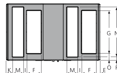
Vue du dessus. Montre les raccords de gaine de la centrale de traitement d'air pour le ventilateur d'air soufflé en bas à droite et en haut à gauche
