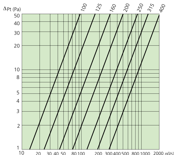
Schéma 1. Débit d'air – Perte de charge SORDO-C 100-400
