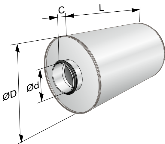
Figure 2. Schéma de dimensions
