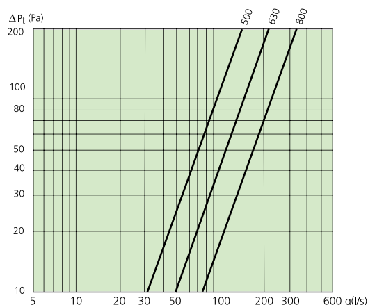
Schéma 2. Débit d'air – Perte de charge SORDO-C 500-800
