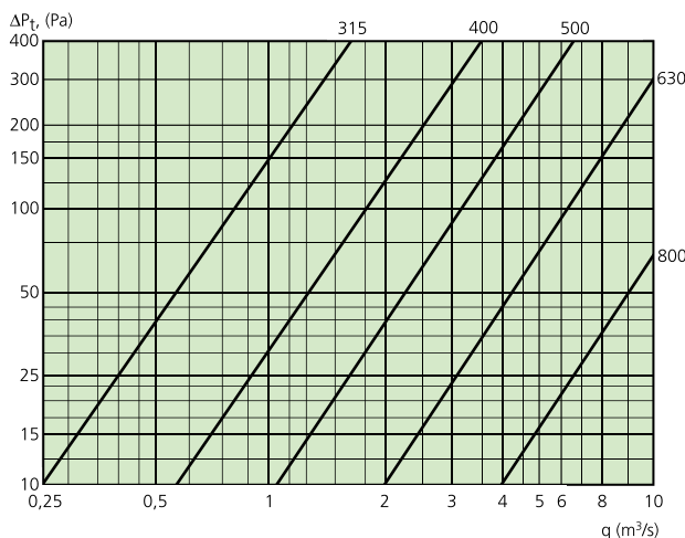
Käyrästä 1. Painehäviö – Ilmavirta
