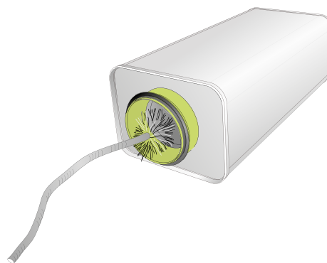
Kuva 2. Ihanteellinen asennus, jossa on suorat kanavat äänenvaimentimen edessä ja takana
