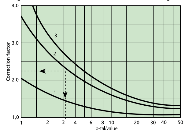
Diagram 1. Korrektion for anden tilslutning
