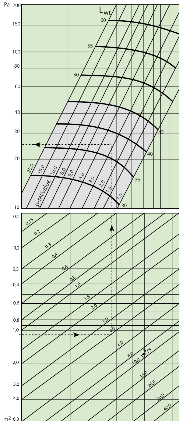
Diagram 1. Korrektion for anden tilslutning
