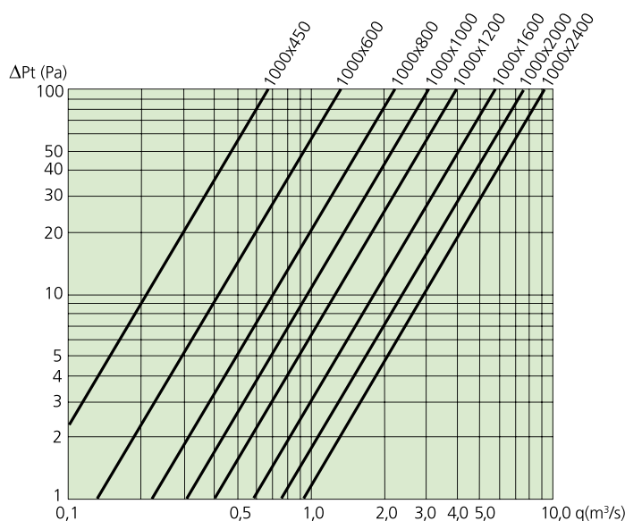
Diagramm 2. ALD Typ 1: Luftvolumenstrom – Druckabfall, (Bruttofläche)
