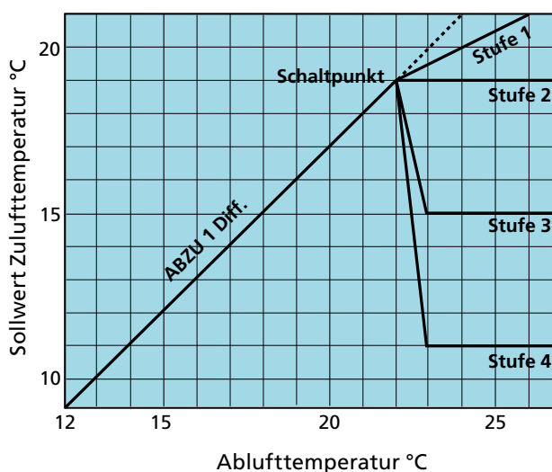
ABZU-Regelung 1, Beispiel
