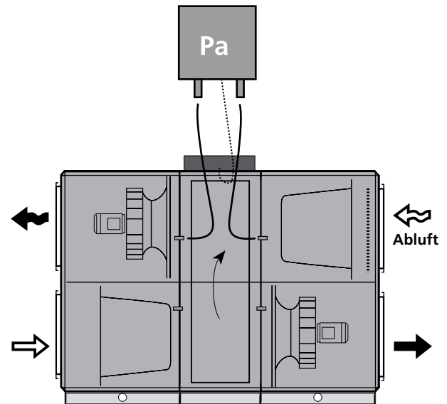
Prinzip der Enteisungsfunktion mit separatem Drucksensor.
