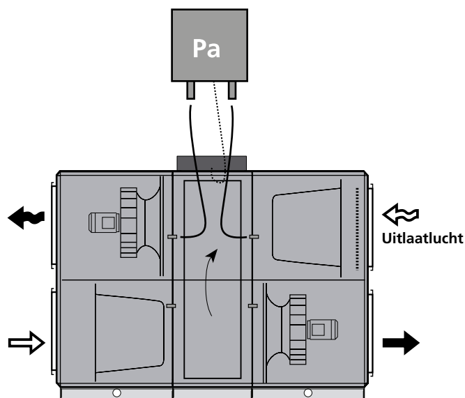
Aansluitprincipe voor de ontdooifunctie met aparte druksensor.
