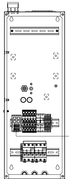
Aansluitkast zonder regelunit (uitlaatlucht)
