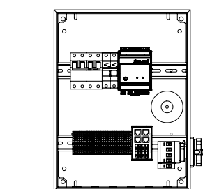
Aansluitkast 809535, pijp-koppeling (accessoire, zie de aparte installatie-instructies)
