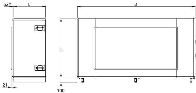
Dimensioni dei raccordi per canali: TCIA 080 1800 x 1000 mm
