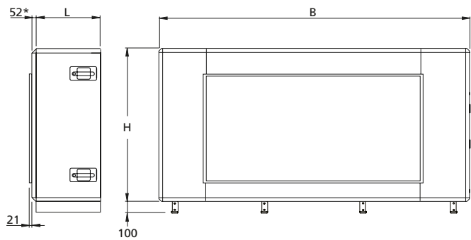
Dimensioni dei raccordi per canali: TCIA 1202.400 x 1.200 mm
