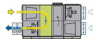
Ricircolo on/off. Ventilatore dell'aria di ripresa arrestato, serrande dell'aria esterna e di quella di espulsione completamente chiuse, serranda della sezione di ricircolo dell'aria completamente aperta.
