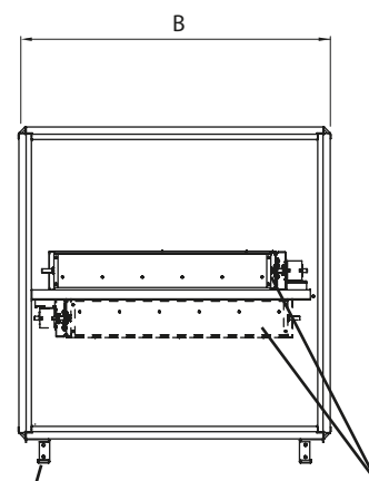
Posizionamento/design del travetto di sostegno, vedere la taglia equivalente dell'unità di trattamento aria GOLD.
