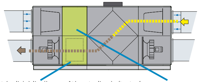
Entrée d'air à l'arrière ou côté porte d'accès (toutes les GOLD PX et GOLD RX 004-040 avec ventilateur d'air extrait au niveau inférieur)
