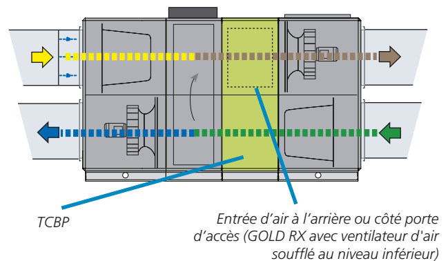
Solutions pour by-pass incendie (arrière, côté inspection ou vers le haut) pour GOLD RX/PX 004-040.
