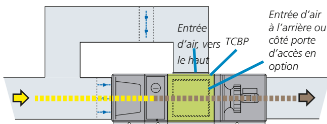
Solution pour by-pass incendie (par le haut, par l'arrière ou côté porte d'accès) pour la centrale de traitement d'air extrait GOLD SD 004-040 en version split.
