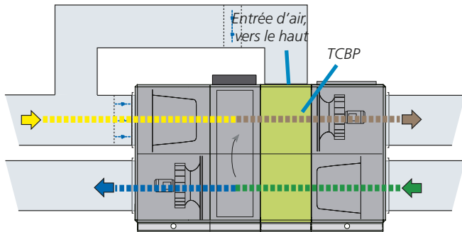
Solution pour by-pass incendie (vers le haut) pour GOLD PX 004-080.
